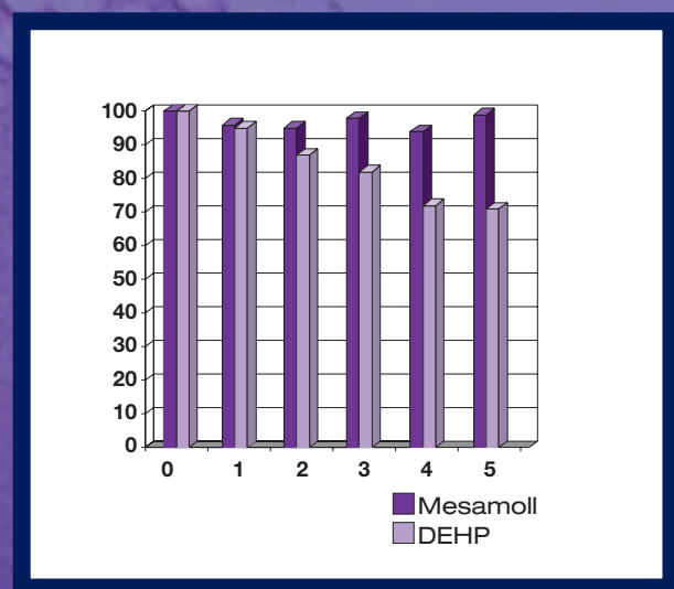
Veränderung der Zugfestigkeit nach Bewitterung im Nordseeklima
